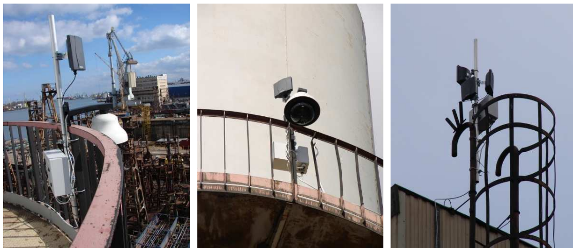
Instalacja systemu monitoringu w Stoczni Gdynia
